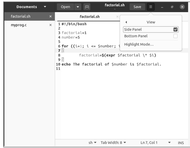
图 10-17 gedit 侧面板
