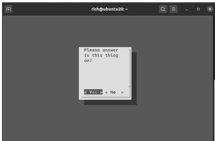
图 18-3 yesno 部件
